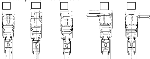
bride: à gauche = côté extérieur / à droite = côté intérieur
